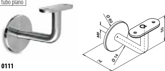
Para tubo plano
