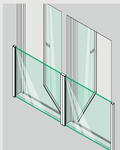
Montaje con perfil intermedio
