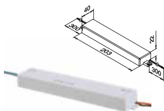
Transformador 12V 220...240V~, CE, sin clavija
