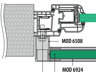
Montaje por delante de carpintería de la ventana
