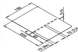
Guía de vidrio
