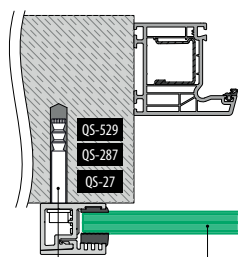
Montaje por delante de fachada
