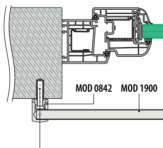
Montaje por delante de fachada
